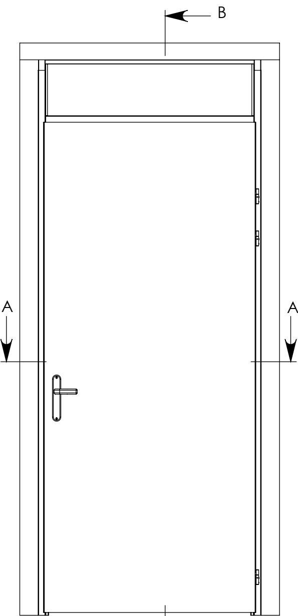
VOORAANZICHT
