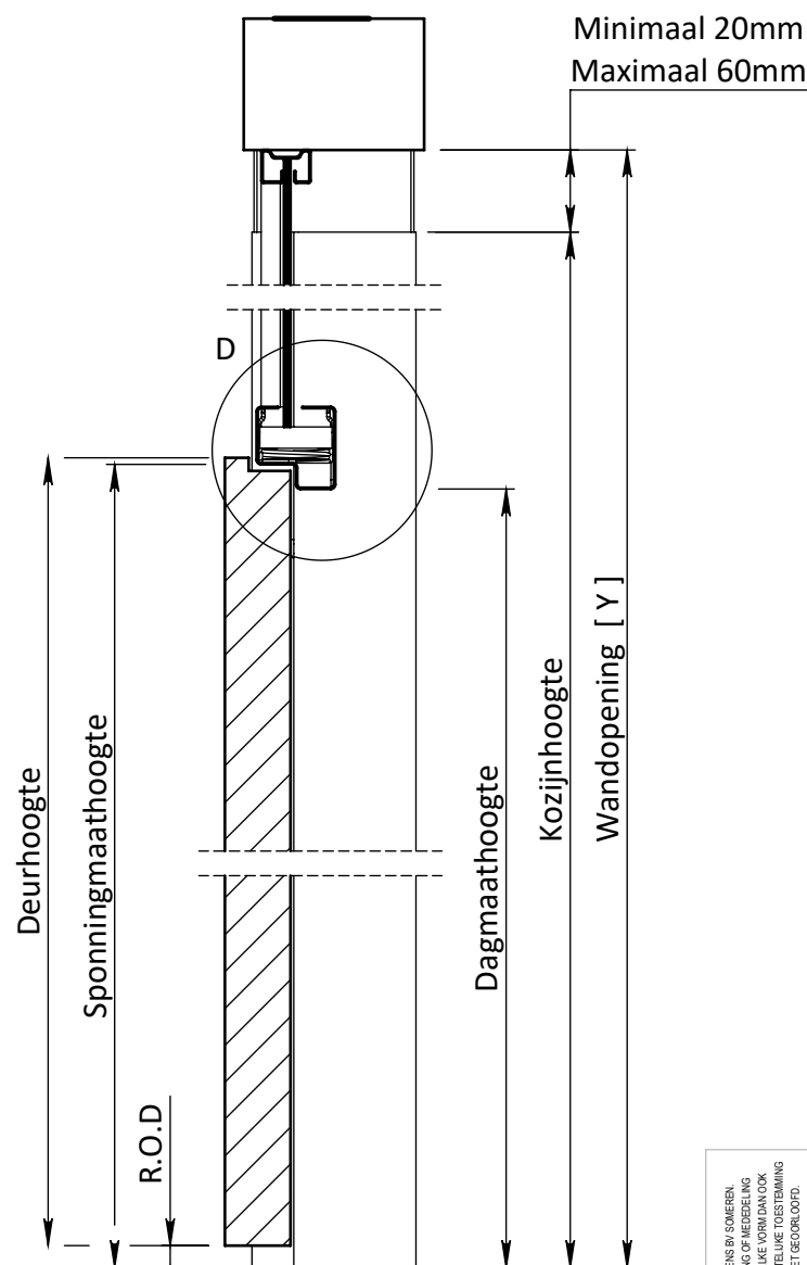
DOORSNEDE B-B
