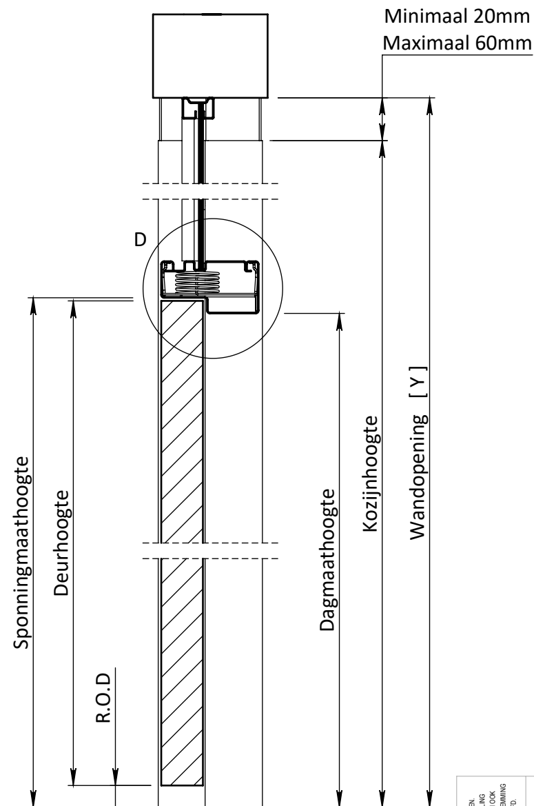
DOORSNEDE B-B
