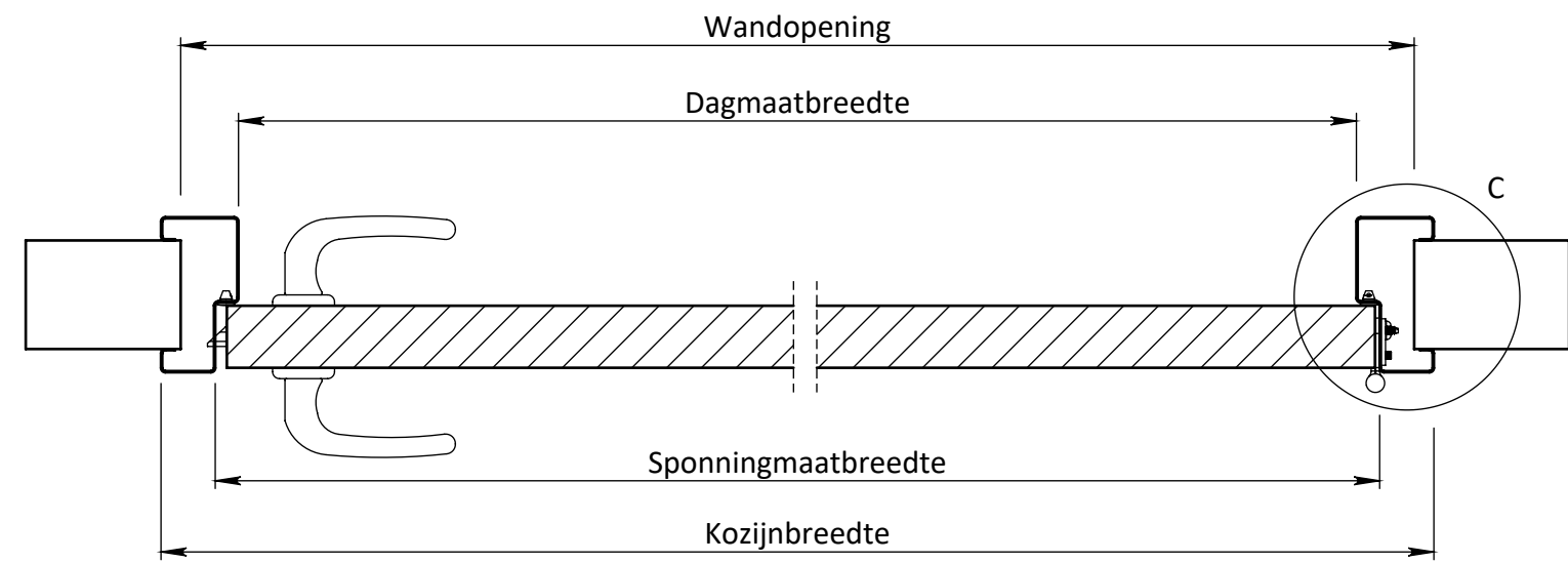
DOORSNEDE A-A
