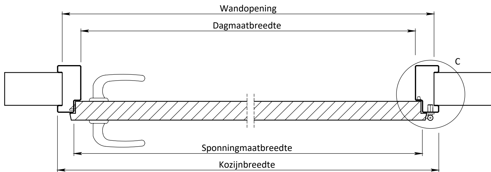
DOORSNEDE A-A
