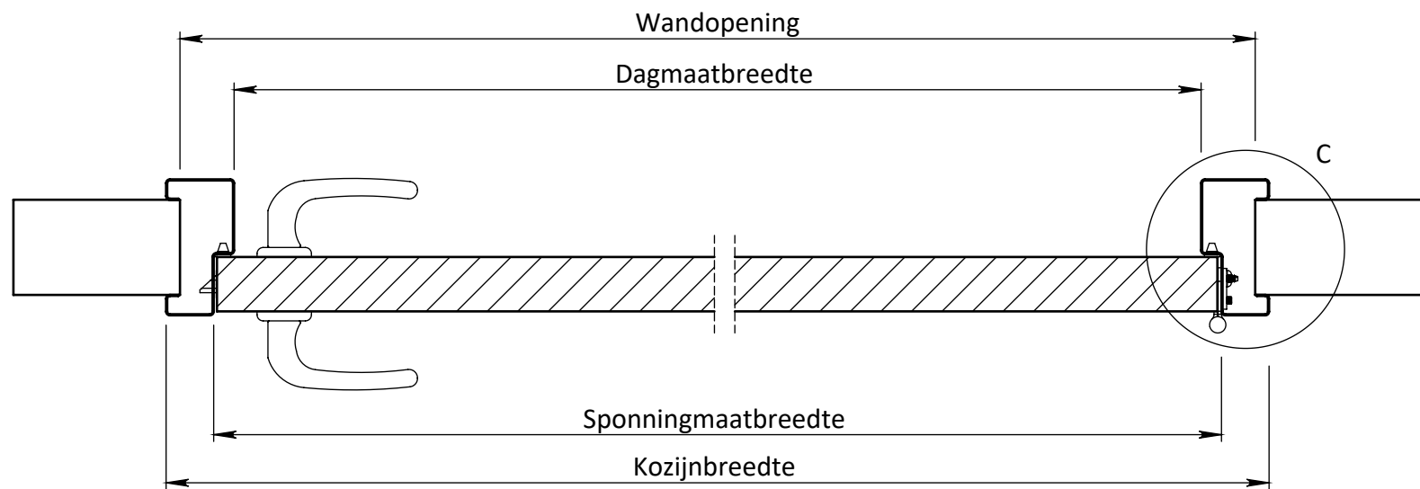
DOORSNEDE A-A
