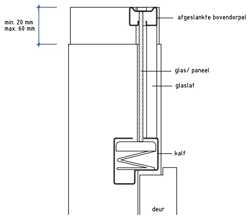
Detail 3: bovendorpel
